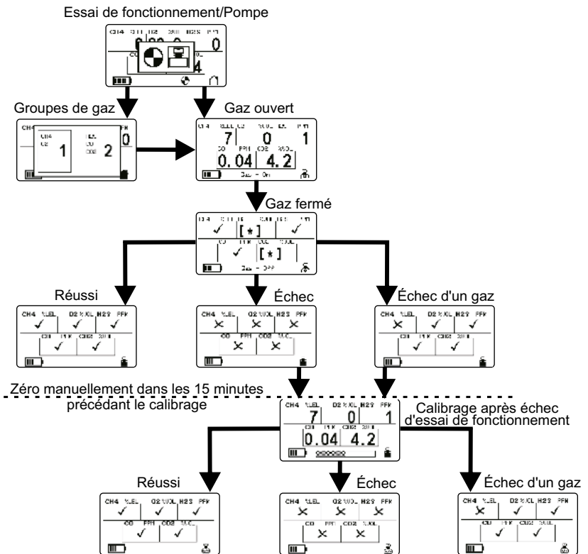
Figure 21: Déroulement des écrans d'essai de gaz
